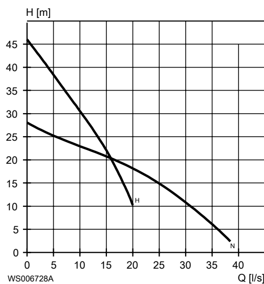
Kuva 14: 50 Hz
