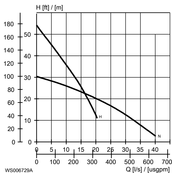
Kuva 15: 60 Hz
