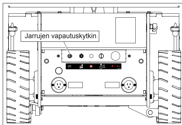
Kuva 6 – Alustan takapää
