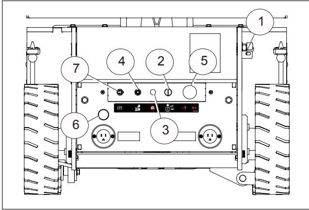
Kuva 2 – Alhaalla sijaitsevat hallintalaitteet alustan takapäässä
