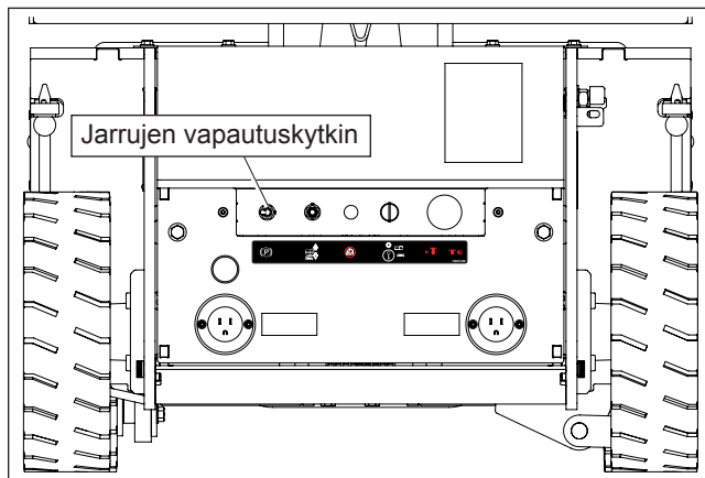
Kuva 8 – Alustan takapä
