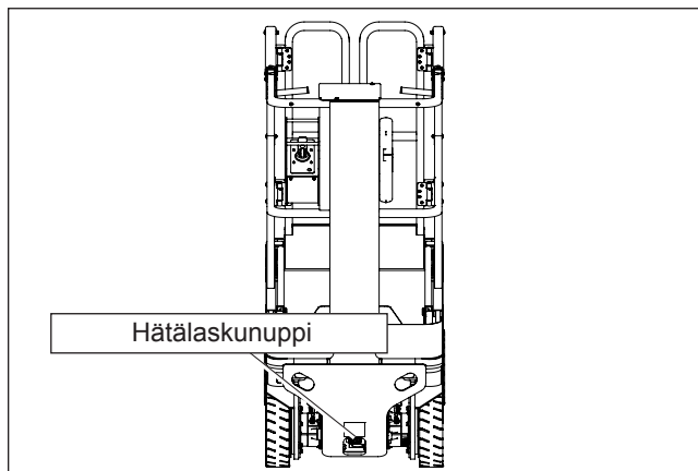
Kuva 5 – Alustan etupää
