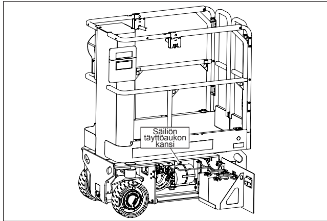
Kuva 11 – Hydrauliöljysäiliö
