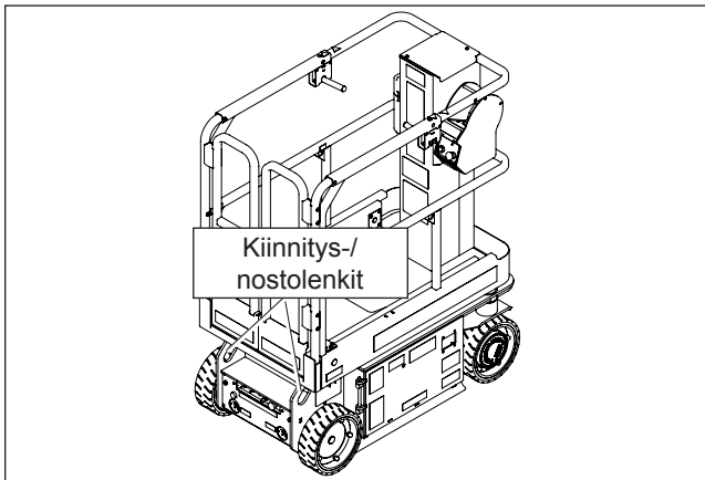
Kuva 10 – Takana sijaitsevat kiinnitys-/nostolenkit
