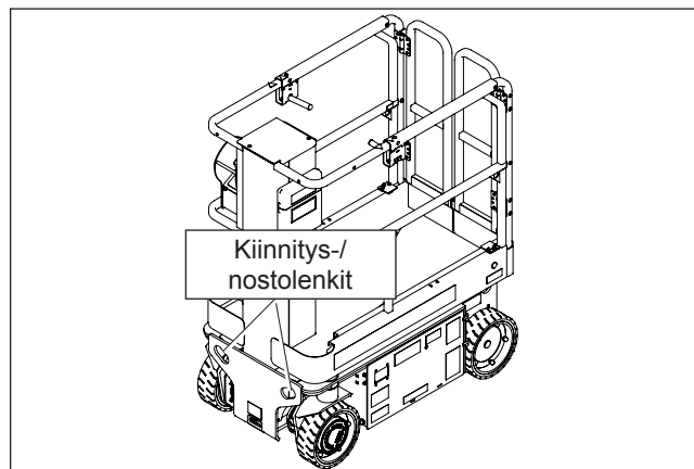
Kuva 9 – Edessä sijaitsevat kiinnitys-/nostolenkit
