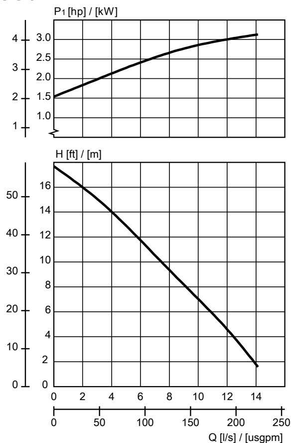
Kuva 13: 60 Hz, 3-vaihe
