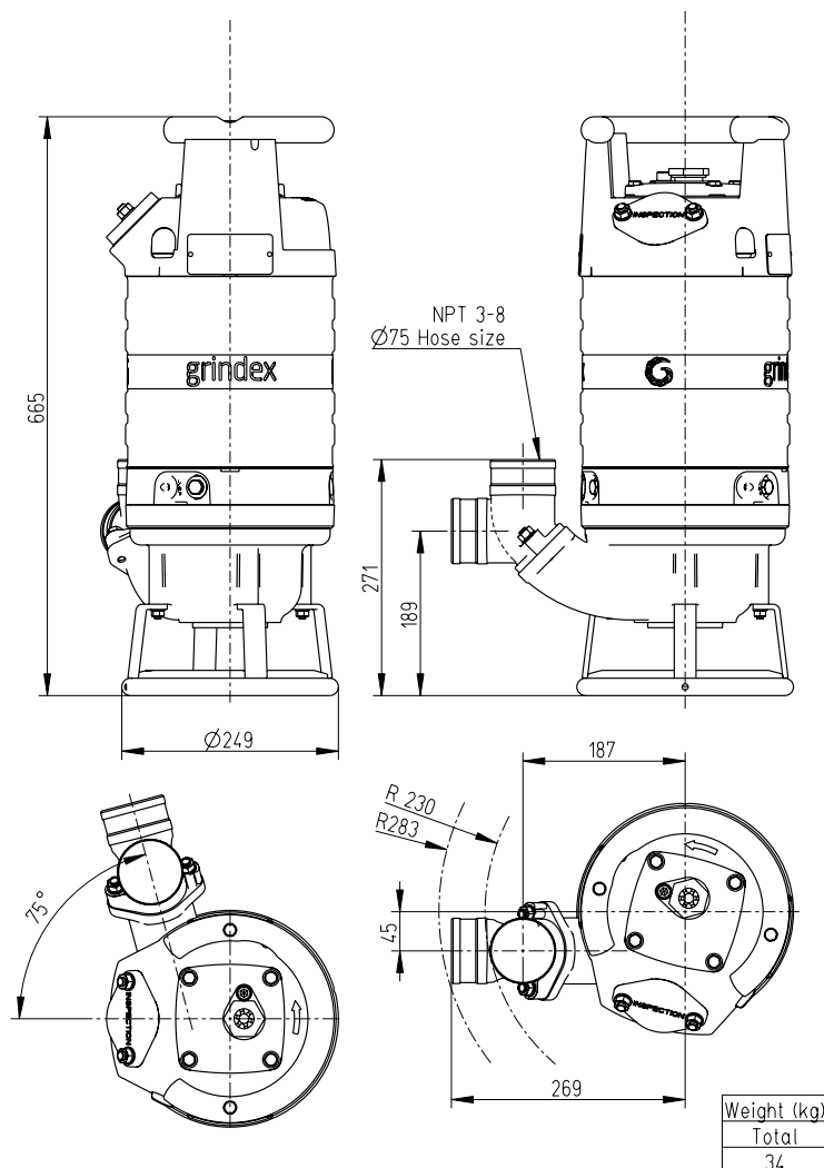
Kuva 10: MSHA-versio
