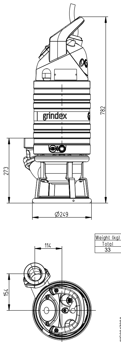
Kuva 9: Vakioversio
